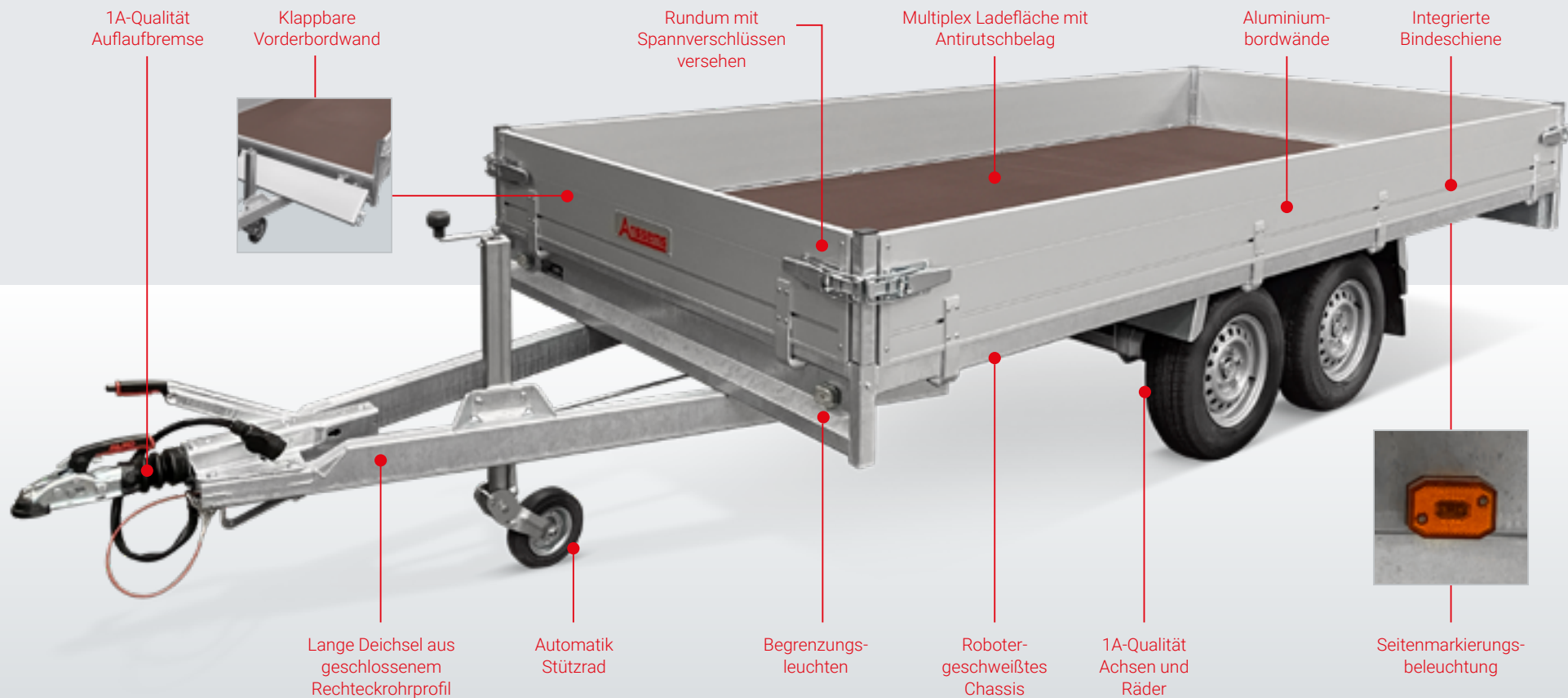
Auffällige Beleuchtung vorne, hinten und an den Seiten
